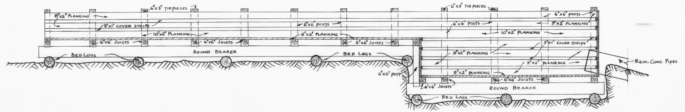
LONGITUDINAL SECTION
