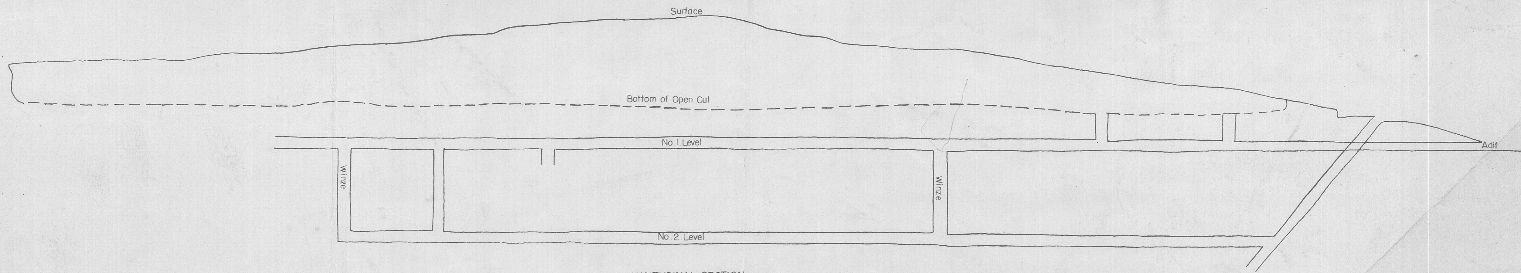
LONGITUDINAL SECTION
