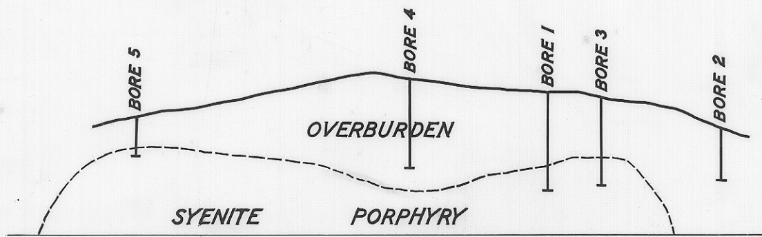
SECTION C-D
