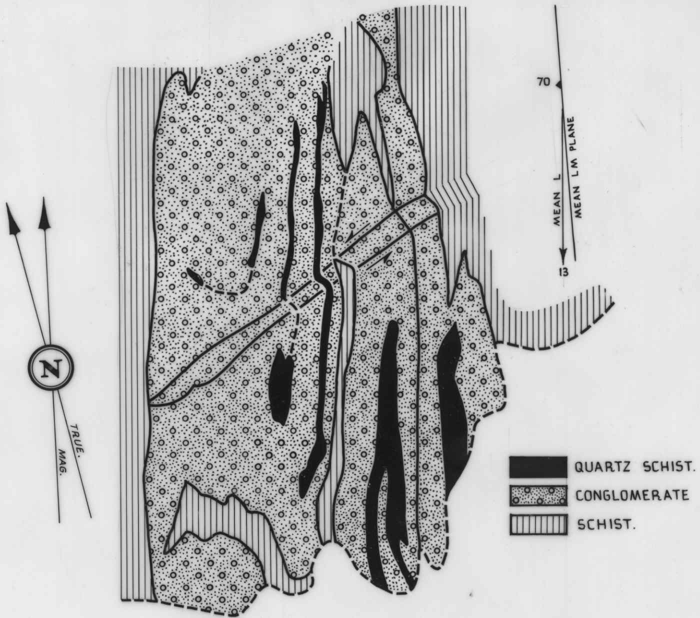
a. PLAN
