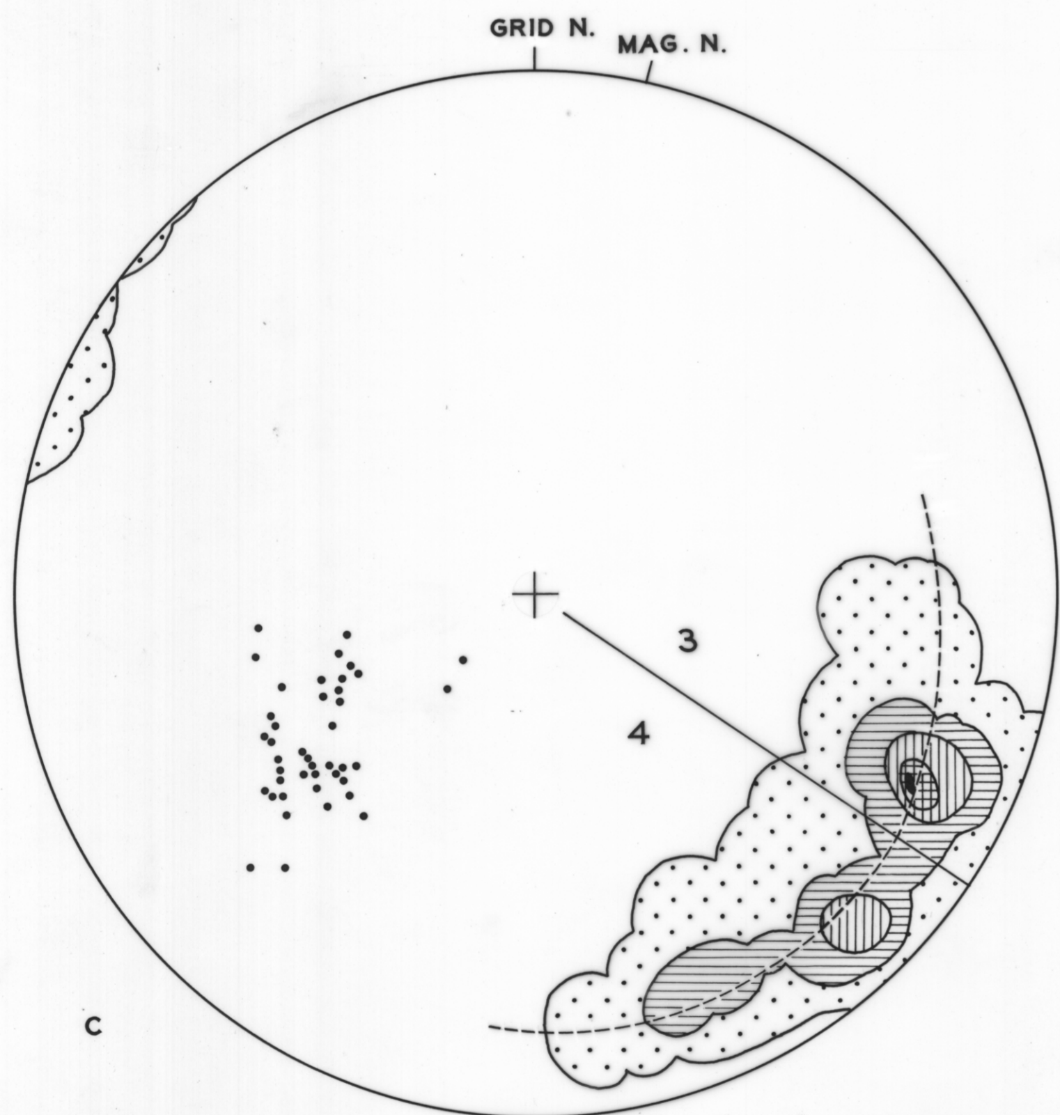
SUBAREAS 3, 4. 50 TS CONTOURS 0-10-20-28-32% SUBAREAS 1-5 • 42ℓ (S 0 S 1 )
