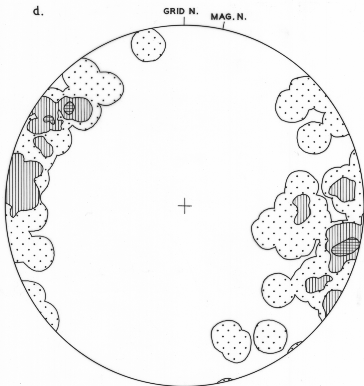
50 FAULTS CONTOURS 0-5-10 %
