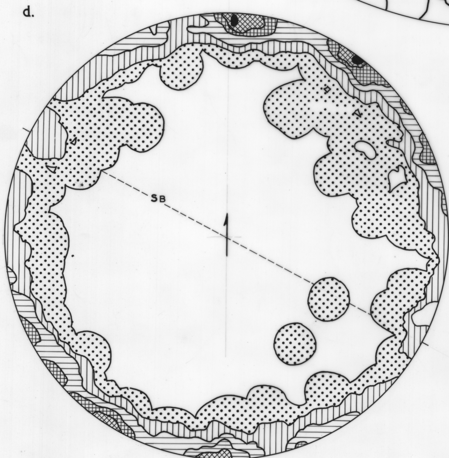
250 MUSCOVITE
