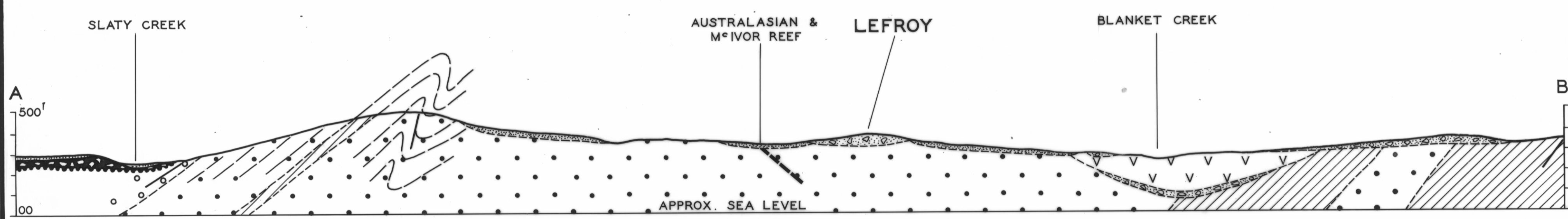
SECTION A-B
