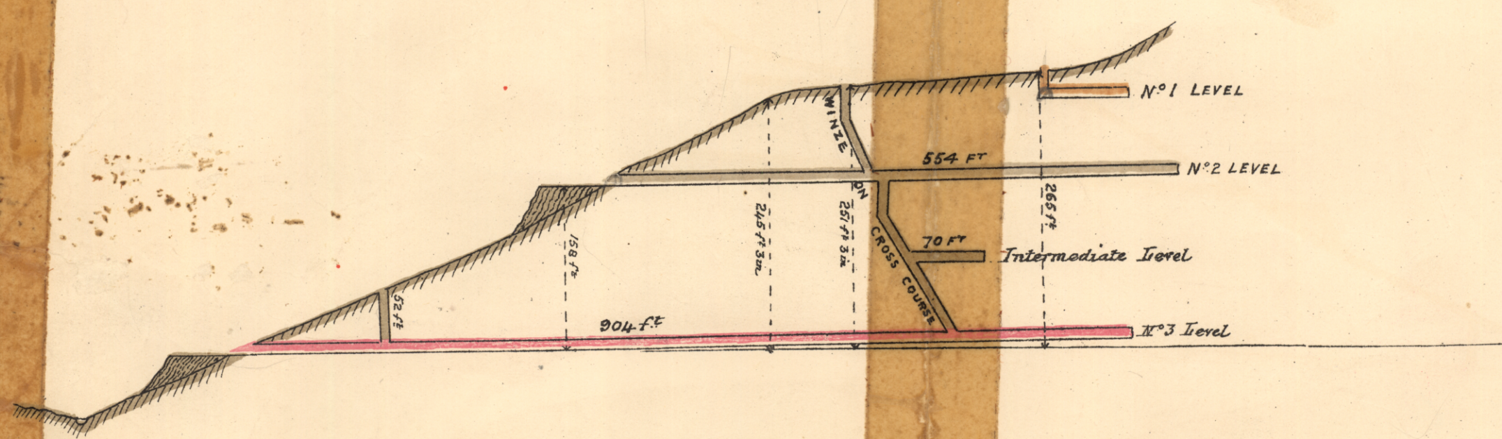
LONGITUDINAL SECTION
