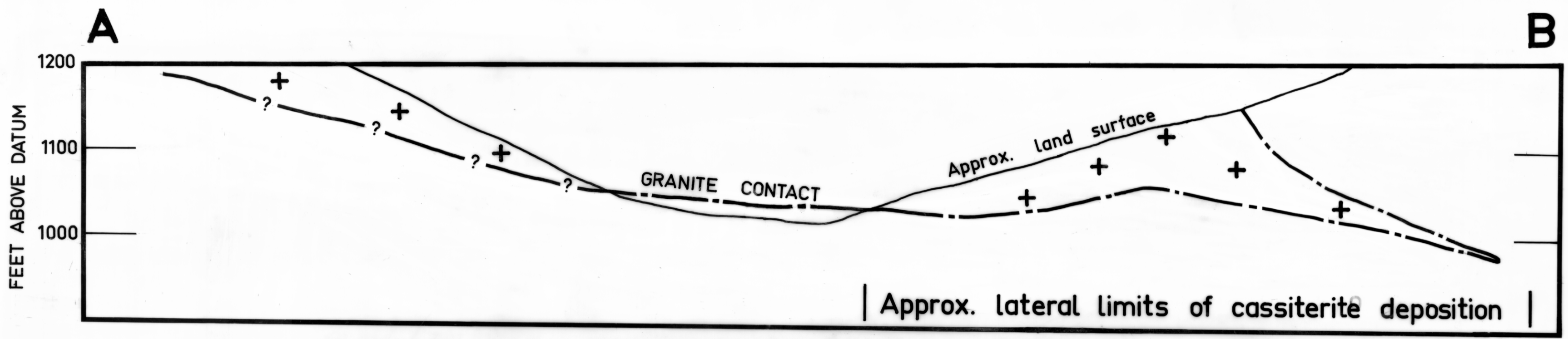
SECTION A-B
