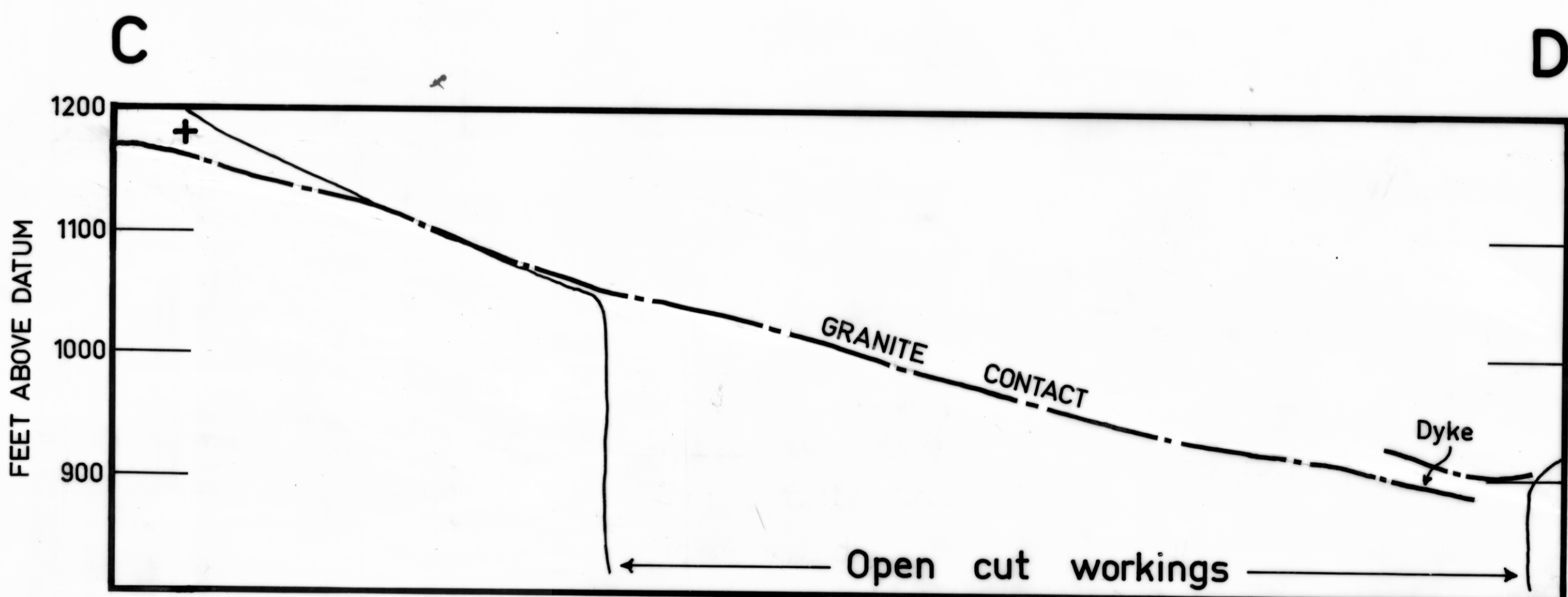
SECTION C-D
