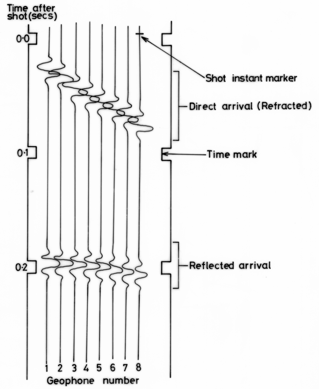
THE SEISMOGRAM
