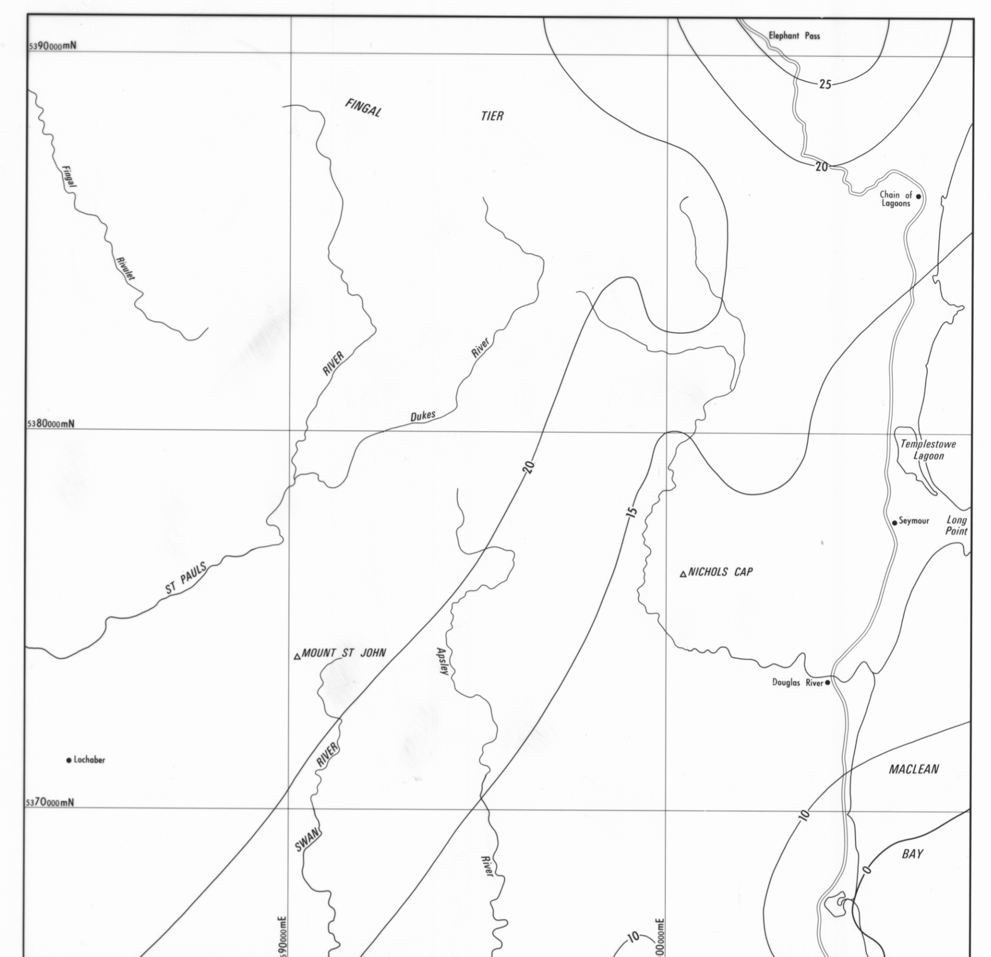
PERMIAN
