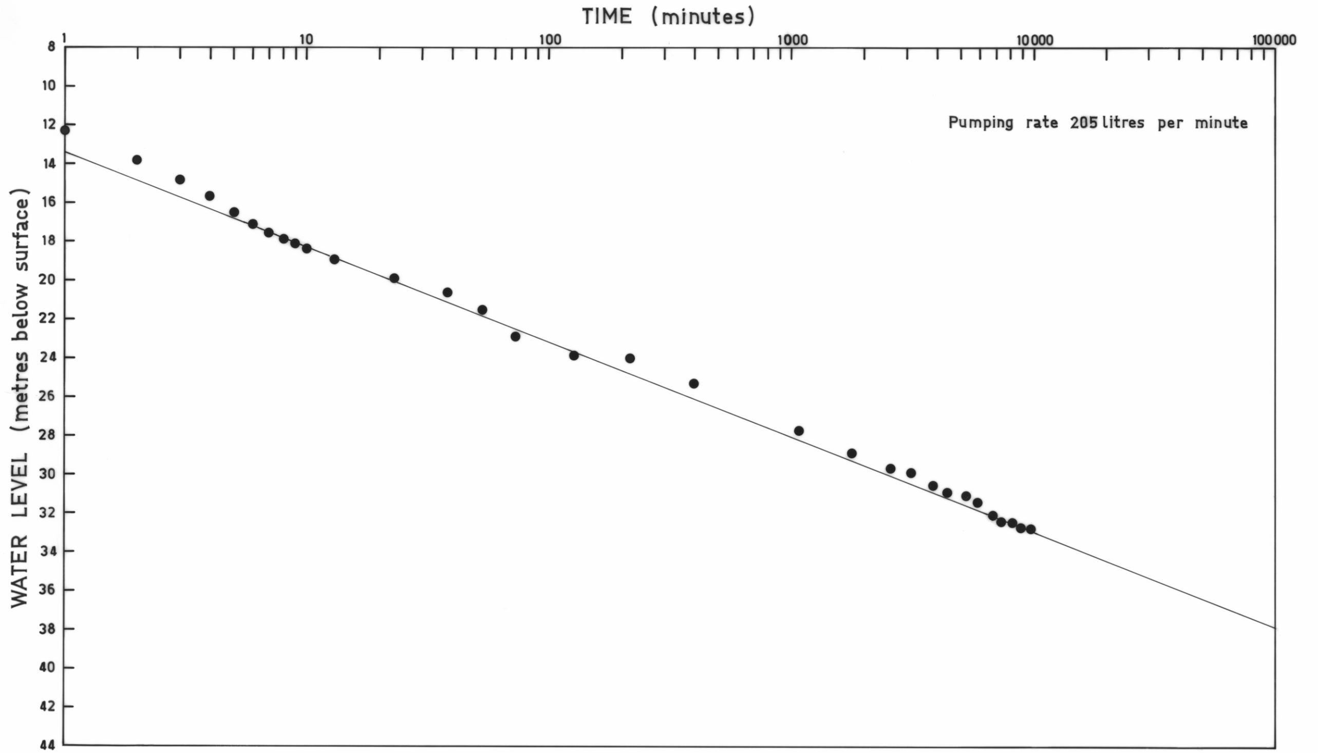
PUMP TEST Nº 3
