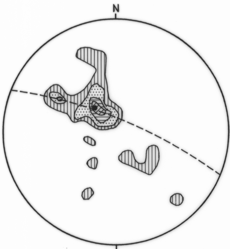
TIPUNAH RD - APIARY RD SYNFORM (CQ540570)
