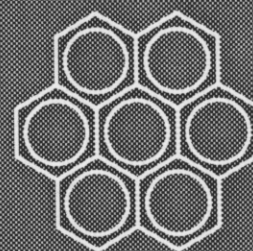
CORONENE
