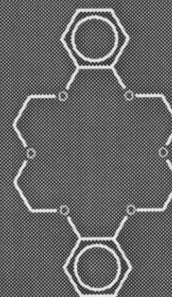
DIBENZO 8 CROWN 6
