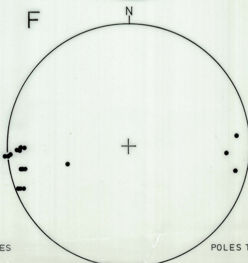
F 1 HINGÉ LINES
