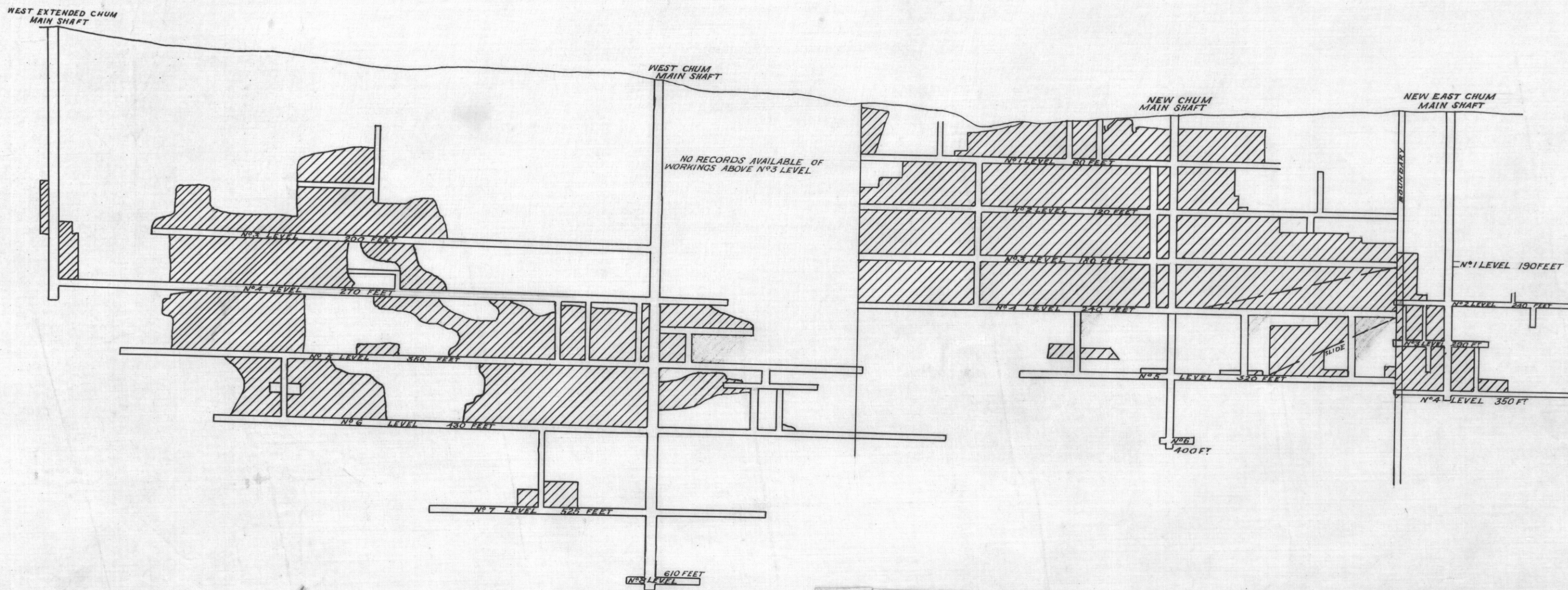
LONGITUDINAL SECTION.
