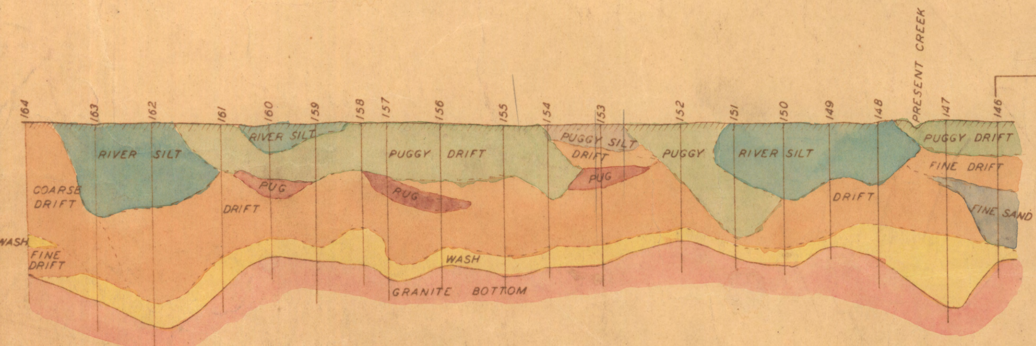
SECTION A-B
