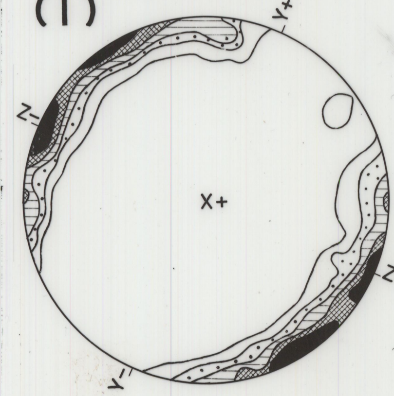
Sl. 6 200 MUSCOVITE 8, 6, 4, 2, 1%
