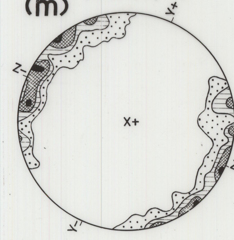
Sl. 7 200 MUSCOVITE 8, 6, 4, 2, 1%
