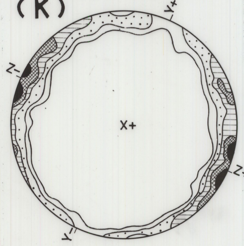
Sl. 4 200 MUSCOVITE 8, 6, 4, 2, 1%
